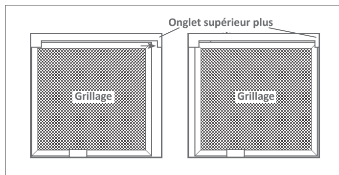
Illustration 11 - Fixation du grillage-moustiquaire
